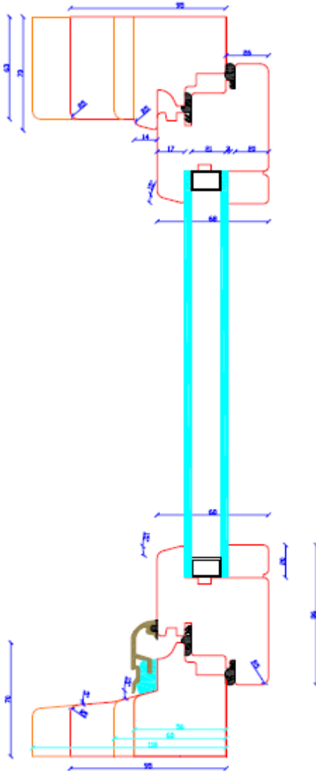
ESCALA 1:2 MARCO 57-120x70-80 HOJA 68x83
