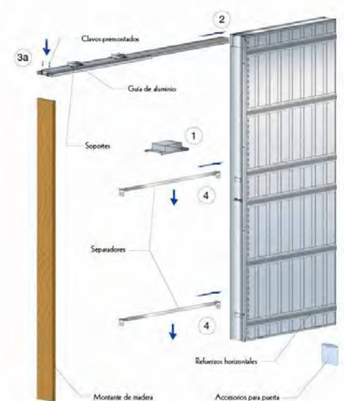
Armazón pladur
