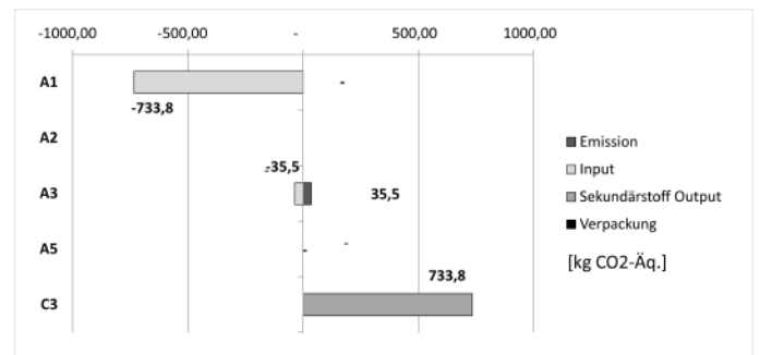
Abb.2: Holzhärente CO 2 -Produktsystemein- und -ausgänge [kg CO 2 -Äq.]. Die inverse Vorzeichengebung der In- und Outputs trägt der ökobilanziellen CO 2 -Flussbetrachtung aus Sicht der Atmosphäre Rechnung.
