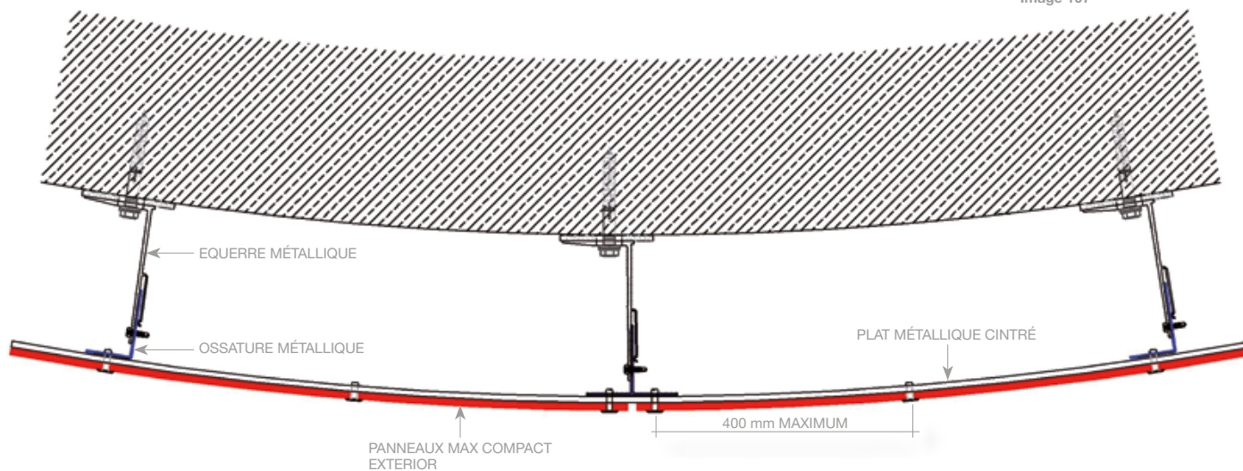
COUPE HORIZONTALE
