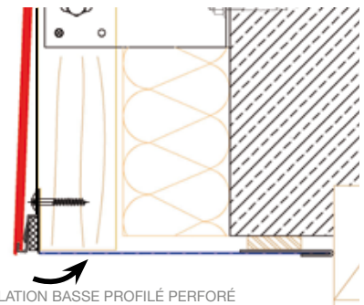
DÉTAIL LINTEAU
