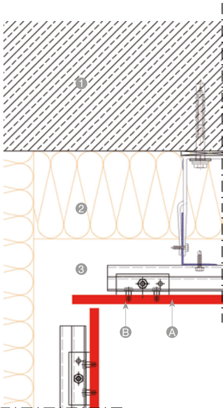
ANGLE RENTRANT
