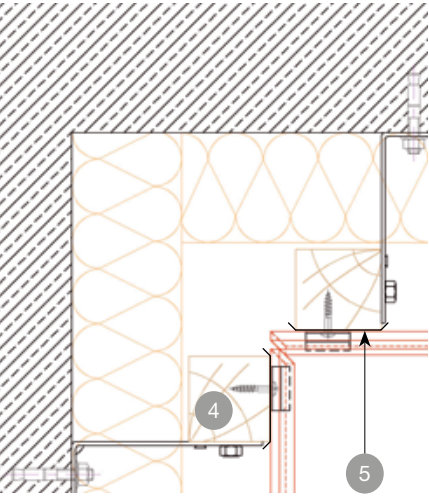
ANGLE RENTRANT
