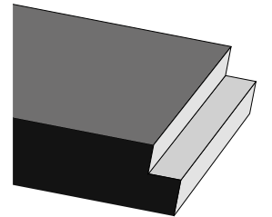
MILLING NOTCH / TYP M
