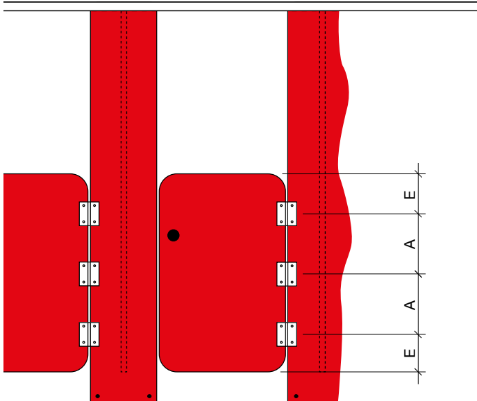
CABINA CON PUERTAS CERRADAS (BISAGRAS CON MUELLES) PARA DUCHAS O RETRETES EN JARDINES DE INFANCIA
