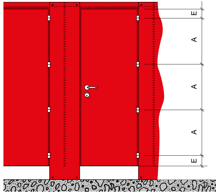
Cabina con columnas Max Compact
