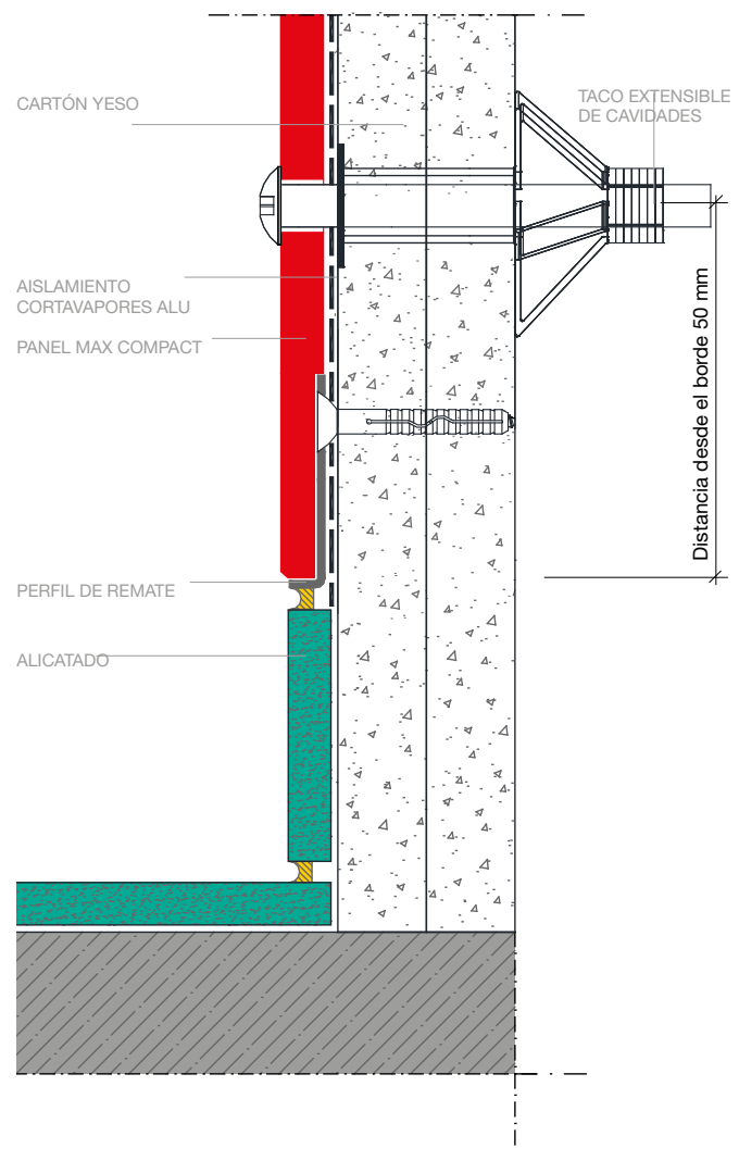
SECCIÓN VERTICAL DE PROTECCIÓN CONTRA IMPACTOS - BORDE INFERIOR AL RAS CON AZULEJO
